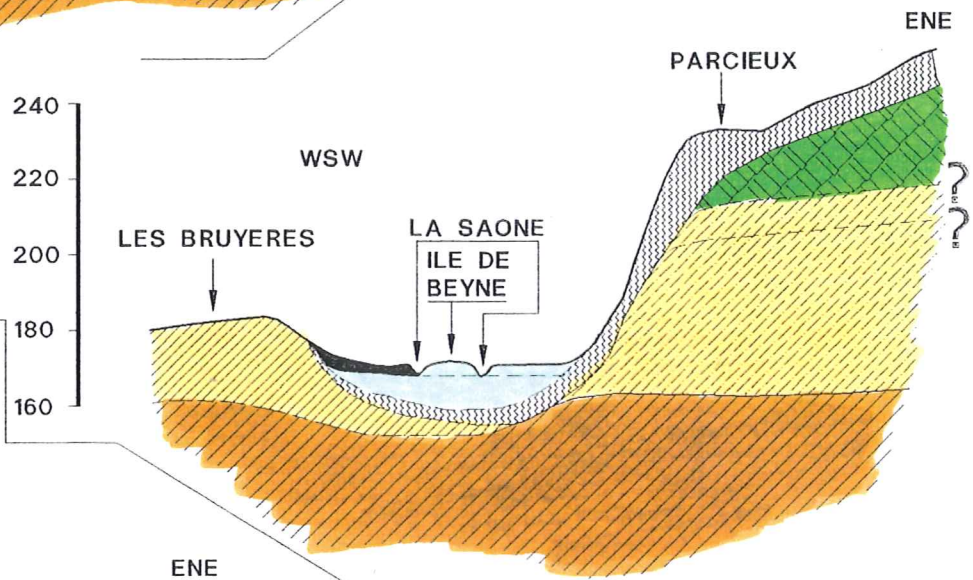
COUPE 45
