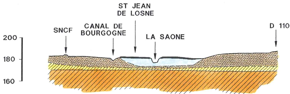
COUPE 22
