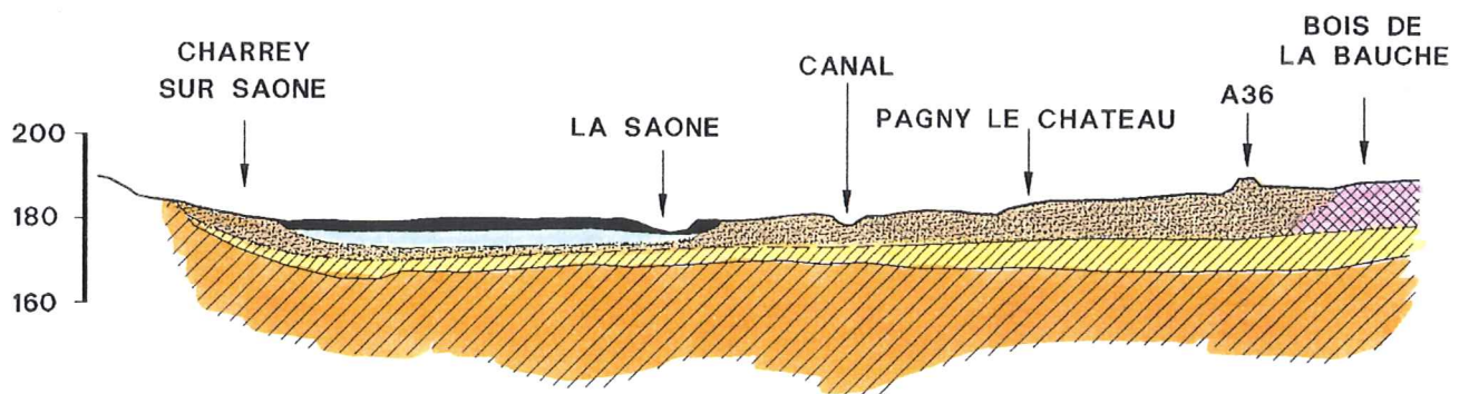
COUPE 23
